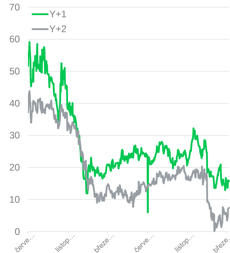
Čistá elektřina (elektřina mínus povolenka) 1 EUR/MWh
