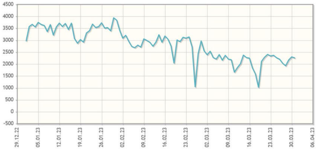
01.01.2023-31.03.2023 PTF Elektrik Fiyatları Ağırlıklı Ortalaması 2.786,28 TL/ MWh
