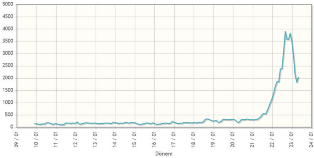
2010-2022/IV. Çeyrek Arası Elektrik Fiyatları Ağırlıklı Ortalamaları (TL/MWh)
