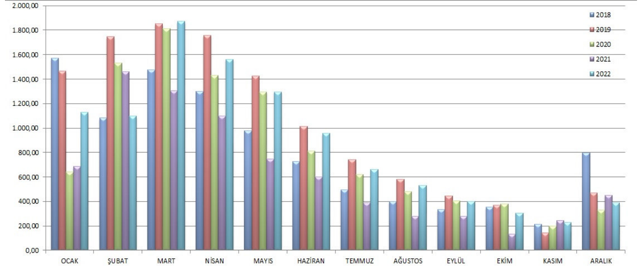
Çukurçay HES- Uzun Yıllar, Aylara Göre Gerçekleşen Üretim Rakamları
