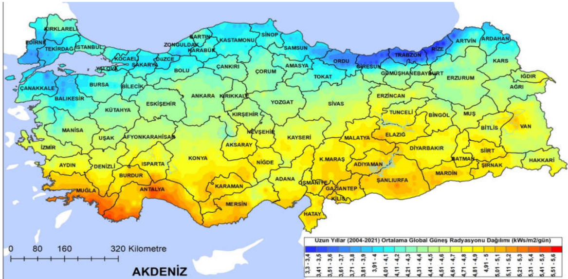
Türkiye Geneli Güneş Radyasyon Haritası ve Işıma Değerleri
