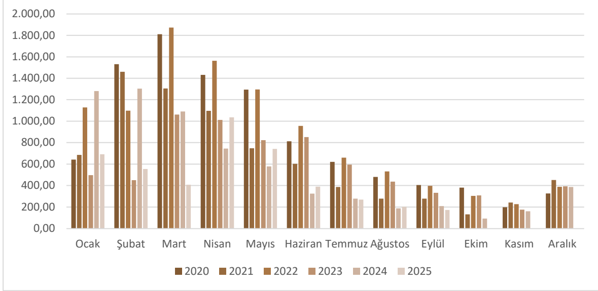
Çukurçay HES- Uzun Yıllar, Aylara Göre Gerçekleşen Üretim Rakamları
