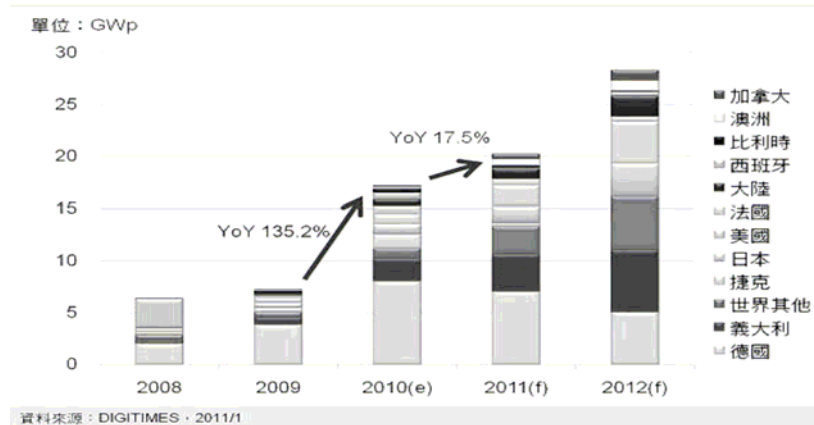
2008~2012 全球太陽光電系統新增安裝量走勢與預估
