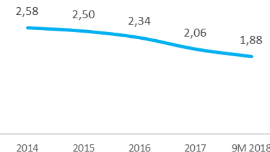
Nettó skuldir/EBITDA
