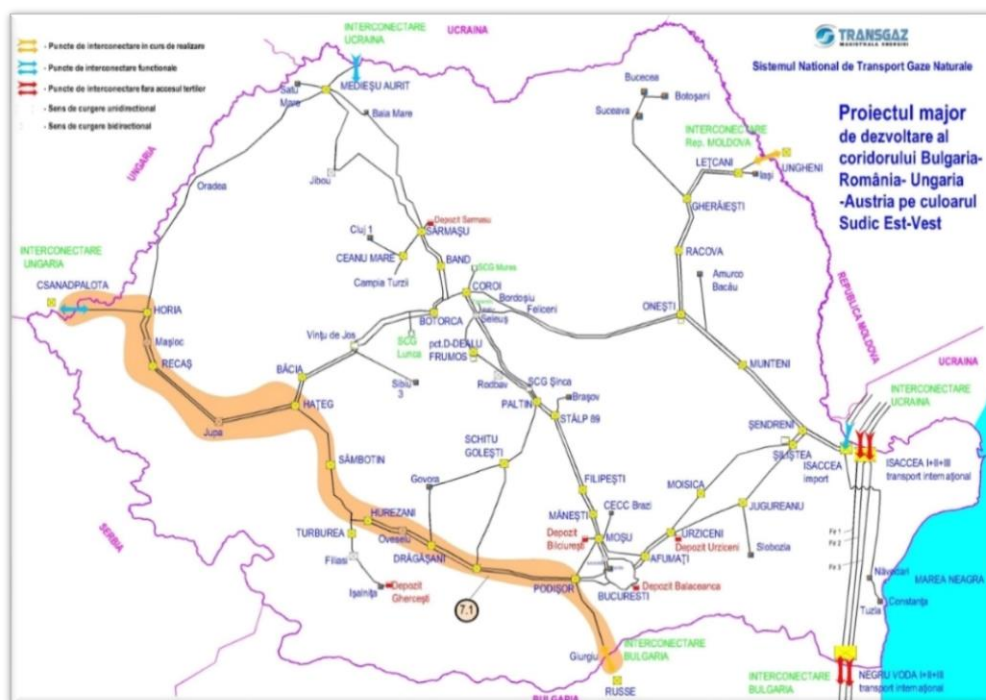
Fig. 2-Coridorul BRUA
