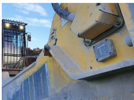
HATCON är en fjärrövervakningsanordning som förbättrar både effektiviteten och säkerheten. På bilden är anordningen monterad på en hydraulhammare (HB 5800).
