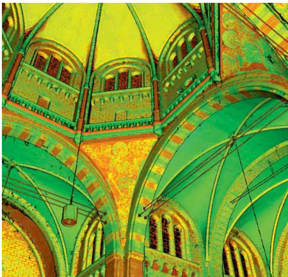
Med hjälp av tredimensionell laserscanning, så kallad High Definition Surveying (HDS), skapades en komplett och precis 3D-modell av kyrkan St Lambertus i Maastricht, Nederländerna. Avbildningen ska användas som underlag vid restaurationen av kulturminnesmärket.
