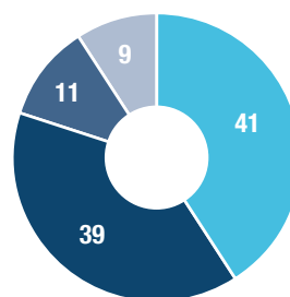
Sveriges elproduktion, %
