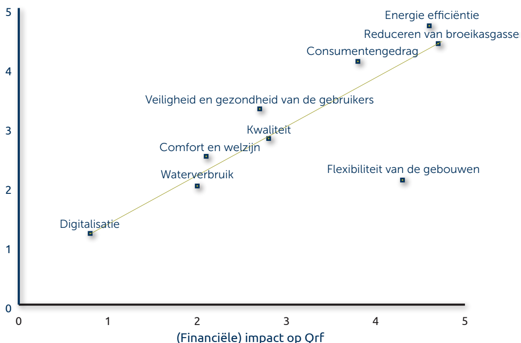
GRAFIEK 1 MATERIALITEITSMATRIX
