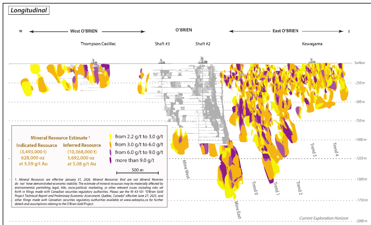
Figure 1 : Le Projet Aurifère O'Brien, de Thompson-Cadillac/O'Brien Ouest, mine O'Brien et jusqu'à O'Brien Est - Vues Longitudinale et en Plan incluant les Ressources Minérales courantes.
