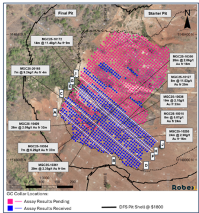
Figure 2 : Emplacements des forages avec contrôle de la teneur sur le gisement de Mansounia pendant les trois premiers mois d'exploitation
