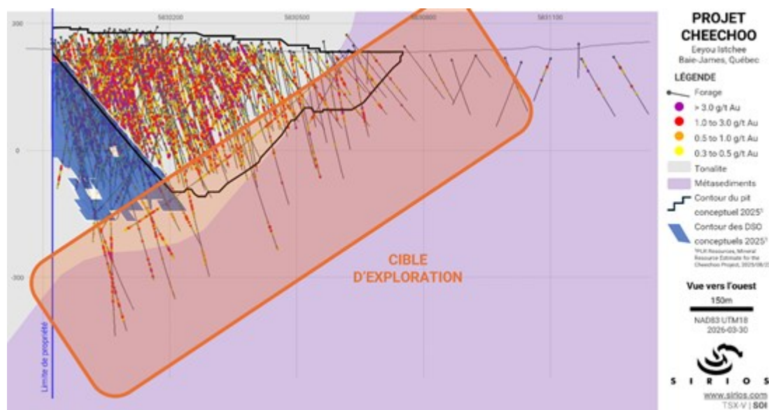
Figure 1 : Cible d'exploration pour le programme de forage proposé de 15 000 m à Cheechoo
