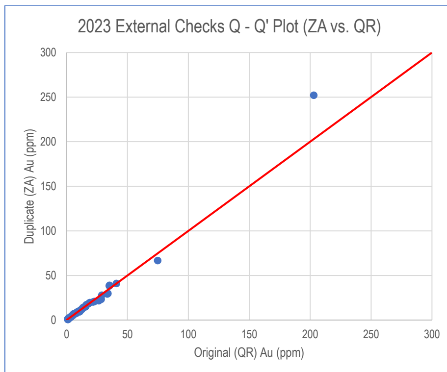
Figure 11-25: Unpaired Q-Q' Plot for 2023 Reject Duplicates (ALS Queretaro vs. ALS Zacatecas) - Gold (g/t)
