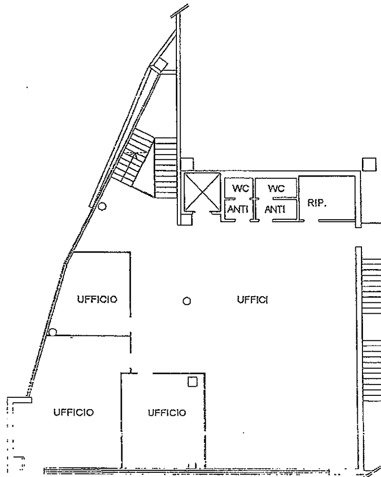
PIANO PRIMO H=3.00m
