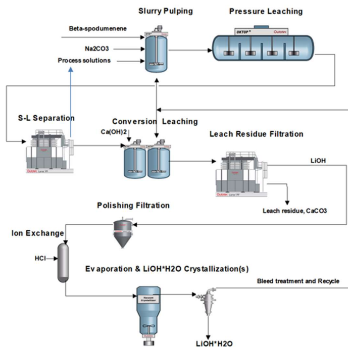
Figure 1 : Organigramme du processus
