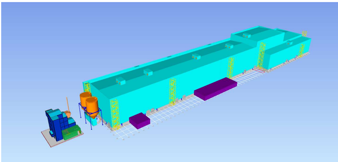
Figure 2 : Vue de l'usine de conversion d'hydroxyde de lithium
