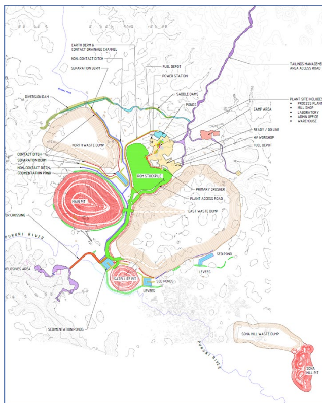
Toroparu Mine Site Layout – Gold X 2019
