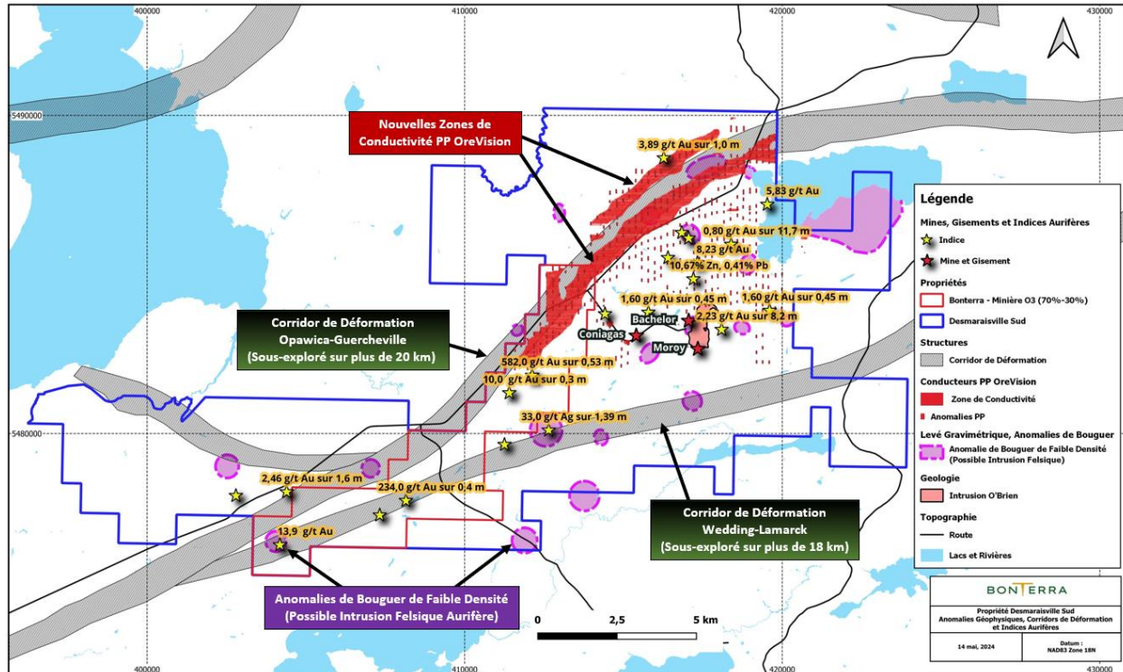
Figure 1- Propriété Desmaraisville Sud, géologie, corridors de déformation et indices aurifères
