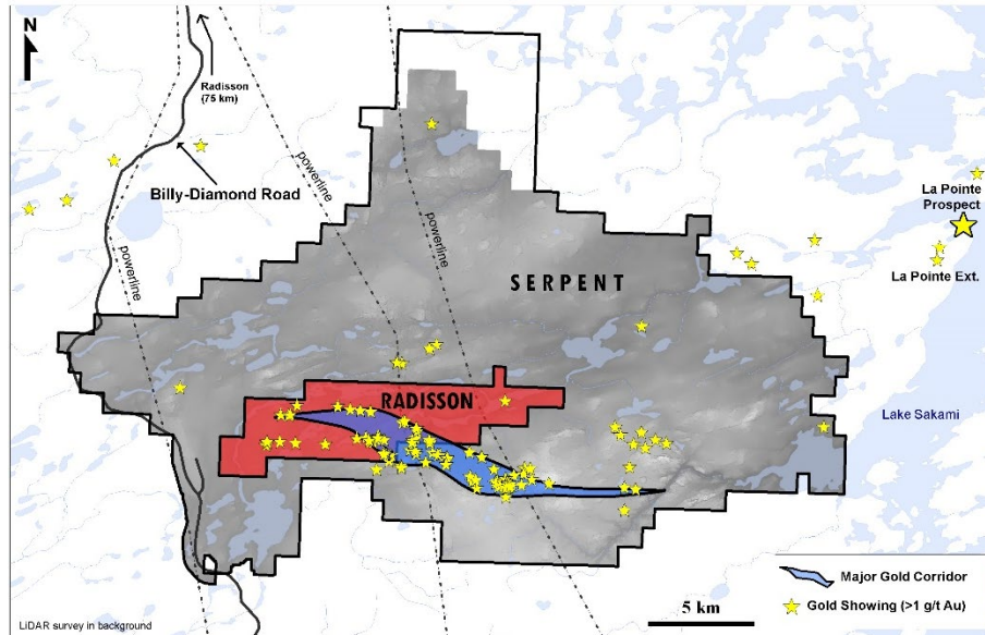
Figure 1. Emplacement du couloir aurifère principal chevauchant la frontière entre les propriétés Serpent et Radisson.
