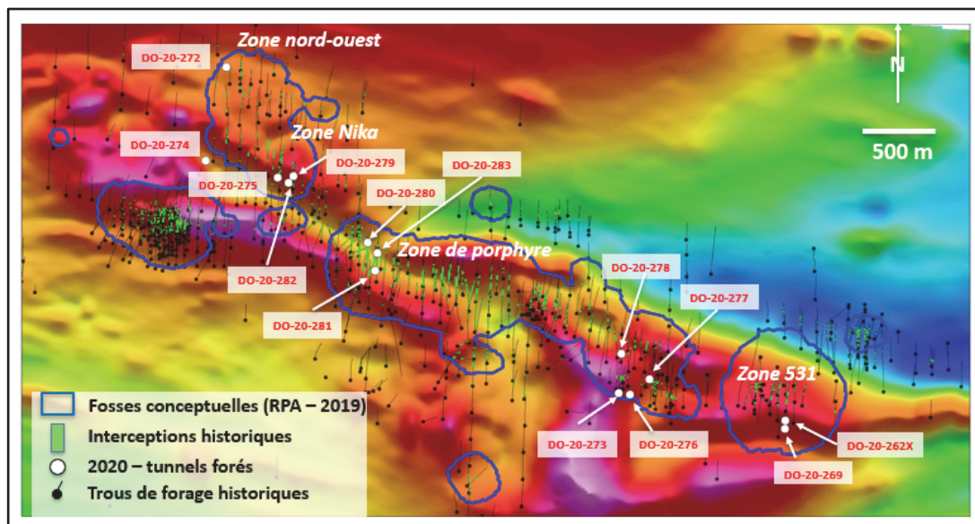
Figure 6 – Interceptions de forage historiques et modèles de fosse Whittle de RPA en 2019. Les sites de forage hivernal de 2020 sont également présentés.
