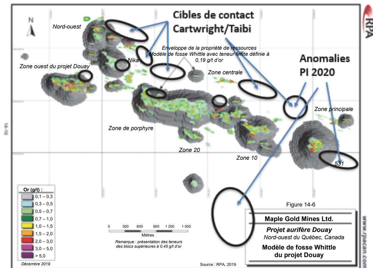
Figure 4 : Étude de base pour les ressources délimitées dans des fosses d'une teneur limite de 0,45 g/t d'or. On remarque plusieurs zones (entourées d'une petite ellipse noire) à teneur plus élevée ayant fait l'objet de forages insuffisants, ainsi que plusieurs lacunes dans le forage entre les zones (plus grandes ellipses). La cible située à l'extrême sud, qui a été définie à l'automne 2020, a été ajoutée à la figure initiale.
