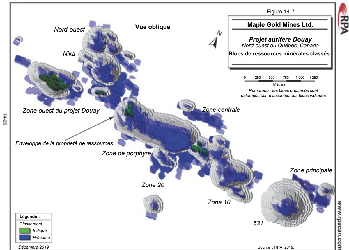
Figure 3 : Blocs indiqués et présumés situés à l'intérieur des limites des modèles de fosse optimisés du projet Douay au 23 octobre 2019, tel qu'il est préparé par RPA. (On remarque que les blocs classés comme présumés sont davantage transparents afin de faire ressortir les blocs indiqués.)
