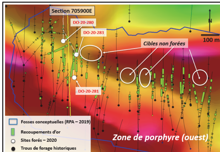
Figure 8 : Plan de forage montrant la répartition des trous de l'hiver 2020 dans la partie ouest de la zone de porphyre. On remarque que le forage est relativement clairsemé le long du côté nord du gisement et que les ellipses blanches indiquent des lacunes de forage plus à l'est.
