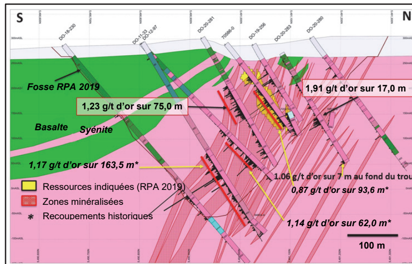
Figure 9 : Section 705900E entre le nord et le sud, avec une vue vers l'ouest, montrant la répartition des trous de l'hiver 2020 par rapport aux trous historiques avoisinants. On remarque une excellente continuité de la minéralisation entre la surface et le fond de la fosse ainsi qu'une minéralisation ouverte sur le côté nord de la fosse conceptuelle actuelle. On remarque également l'étendue limitée des ressources indiquées compte tenu du forage clairsemé au moment de la mise à jour de l'estimation des ressources (soit vers la fin de 2019), avant les forages réalisés en 2020.
