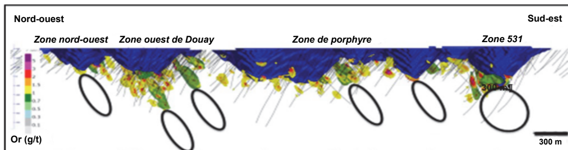
Figure 5 : Vue longitudinale verticale de la section nord-ouest et sud-est (toutes les zones) montrant la répartition des blocs souterrains sous la fosse dont la teneur est supérieure à la teneur limite de 1 g/t d'or.
