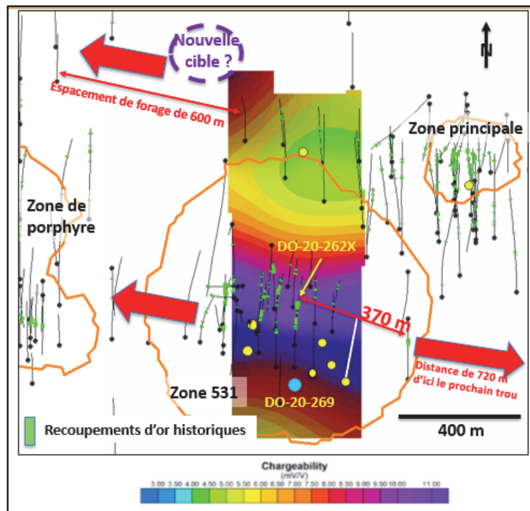
Figure 11 – Résultats des lignes de PI tridimensionnelle (chargeabilité) pour l'hiver 2020, présentés selon une vue en plan (tranche de profondeur de 450 mètres) pour la zone 531. On remarque la chargeabilité de la zone 531 qui est ouverte vers l'est-sud-est et l'ouest-nord-ouest, ainsi que la nouvelle cible dans l'extension ouest-nord-ouest de la zone principale.
