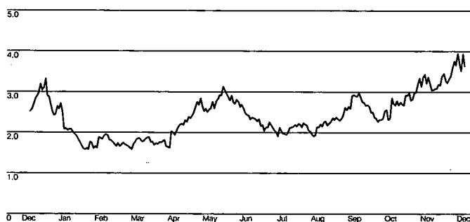
Henry Hub natural gas price 2024 $ per mmBtu
