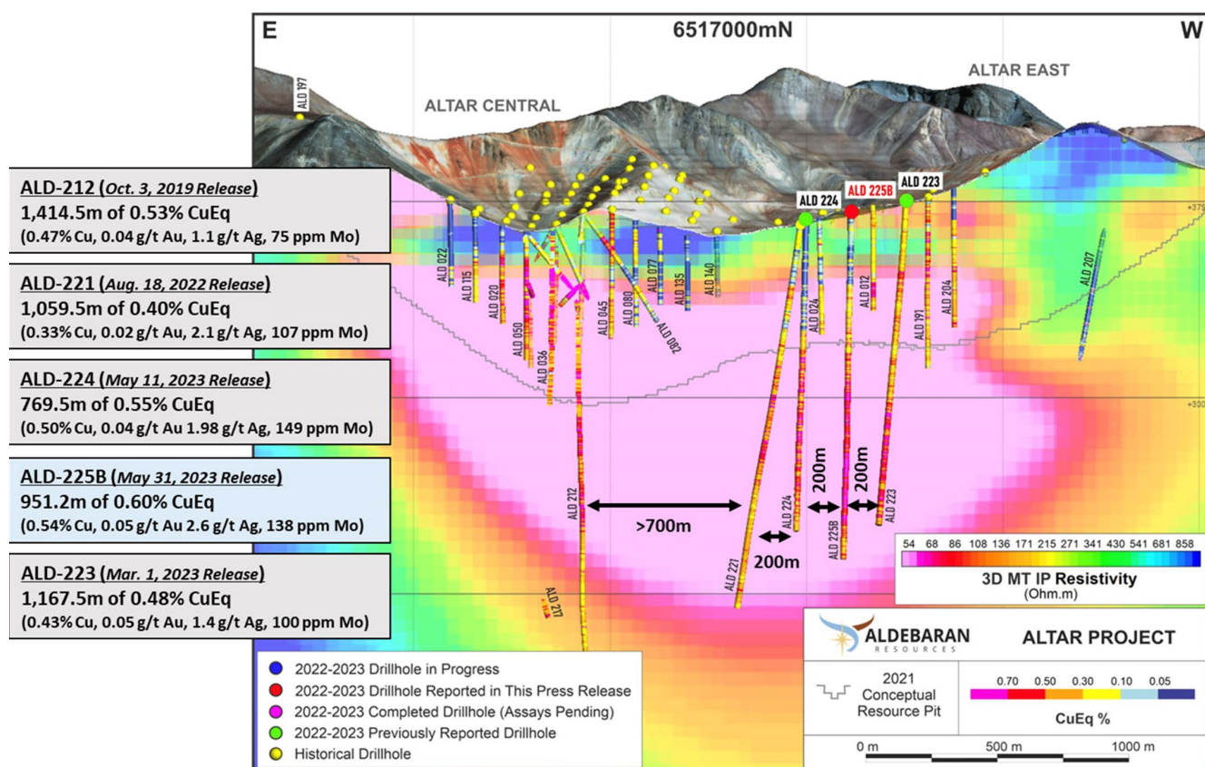
Figure 4 : Coupe transversale en direction du nord-est
