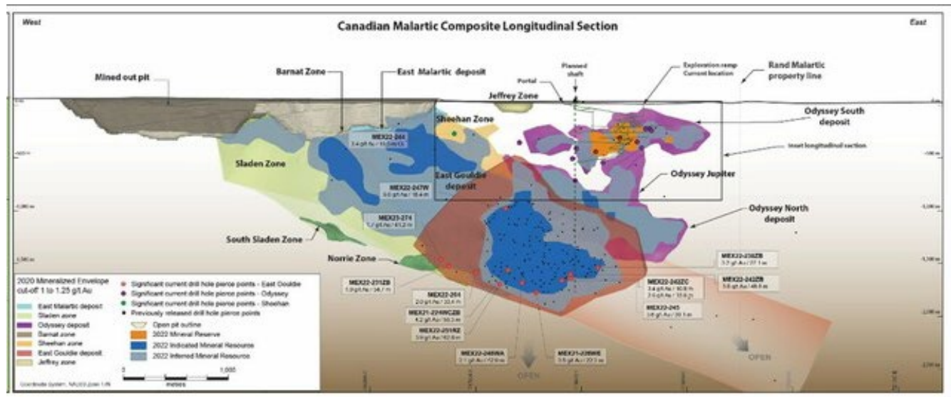
Figure 2 : Section longitudinale de Canadian Malartic
