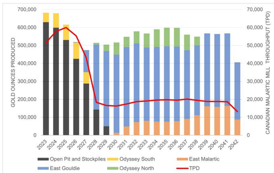
Figure 1 : Profil de production de Canadian Malartic
