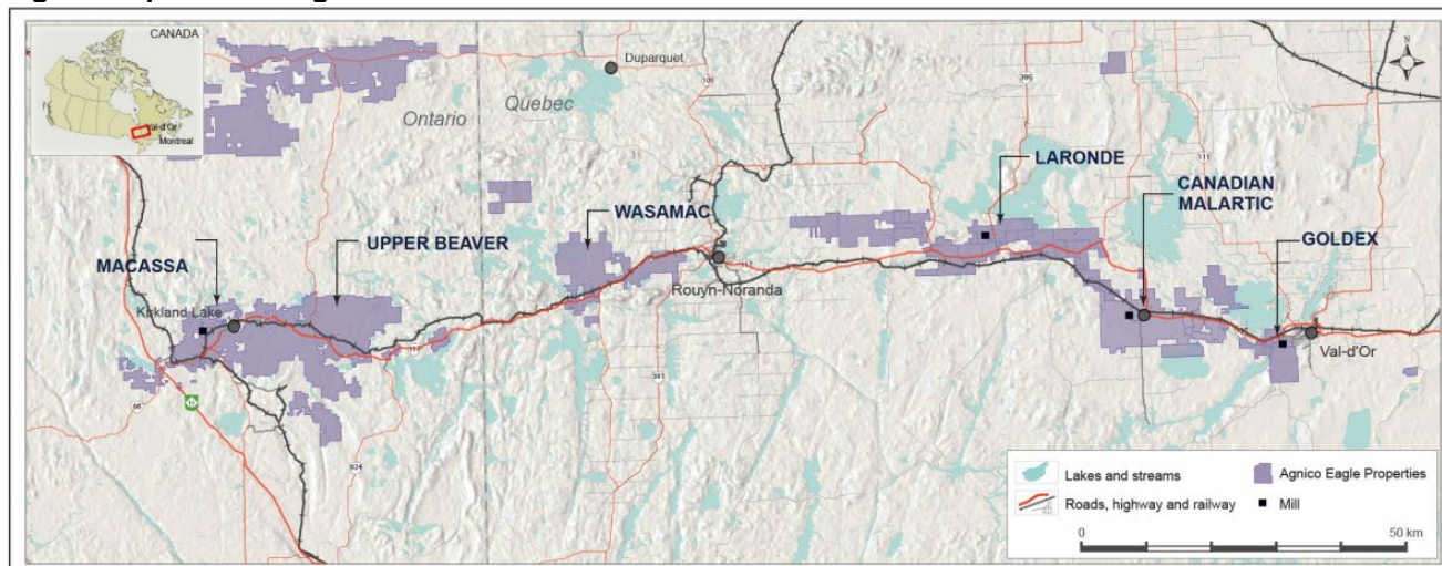
Figure 3 : présence régionale – faille Cadillac-Larder Lake
