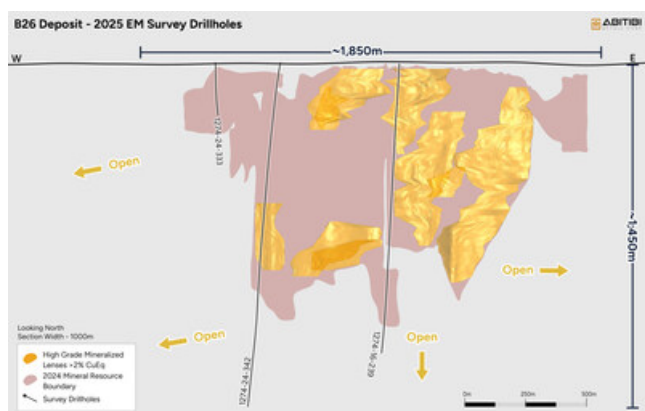
Figure 1: Downhole EM Pulse Survey (CNW Group/Abitibi Metals Corp.)
