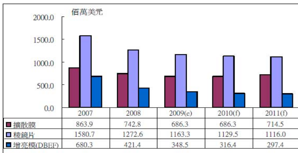
圖二 2007~2011 全球 LCD 光學膜生產規模趨勢分析
