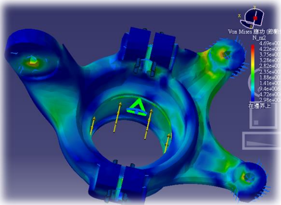
2. 可行性評估 FEA & Grain Flow simulations
