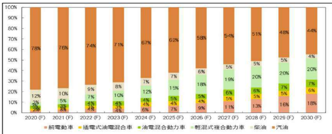
全球未來 10 年輕型車銷售占比(依動力系統分類，圖例順序由下到上)
