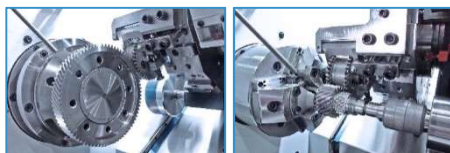
毛邊去除機構
