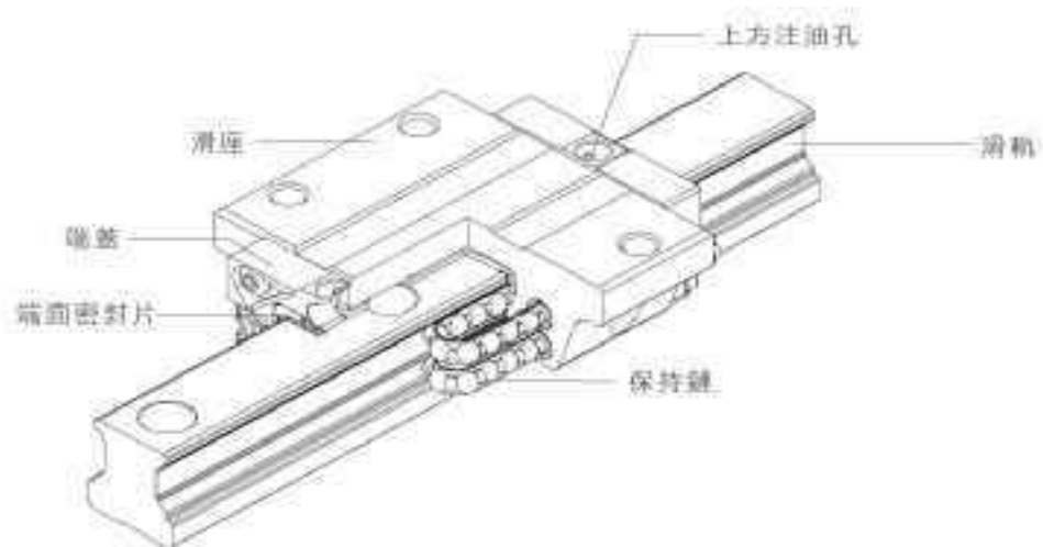
線性滑軌示意圖
