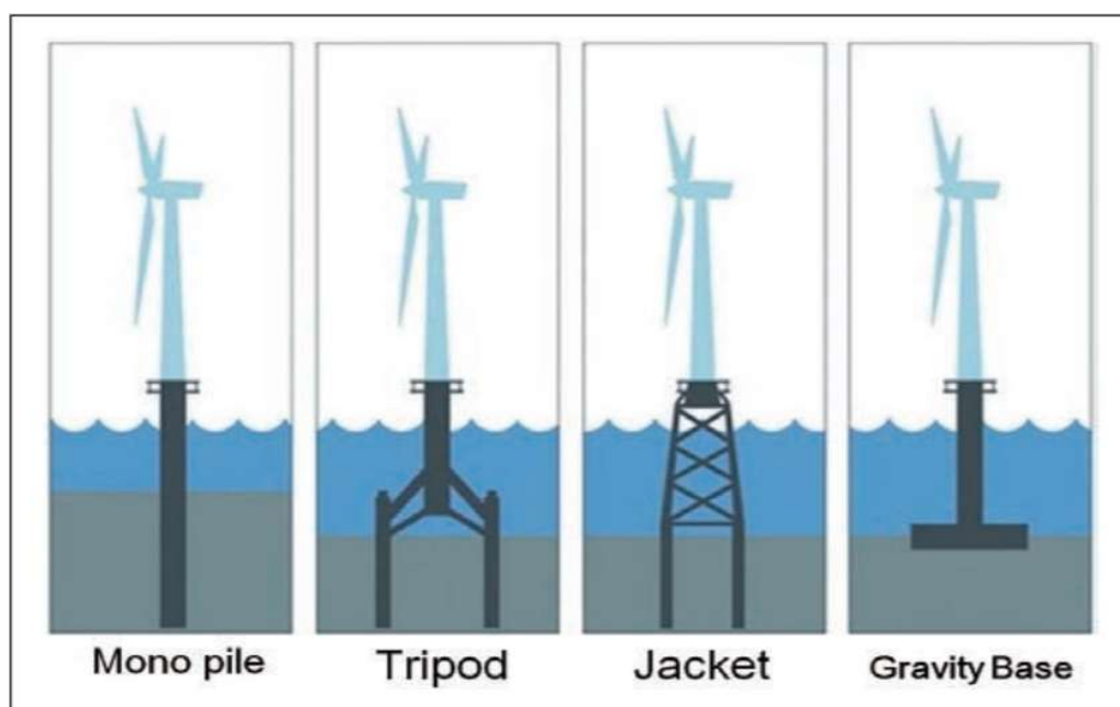
【離岸風電水下基礎型態】
