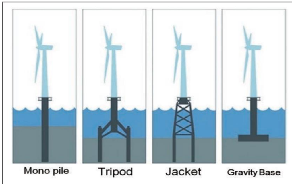
【離岸風電水下基礎型態】
