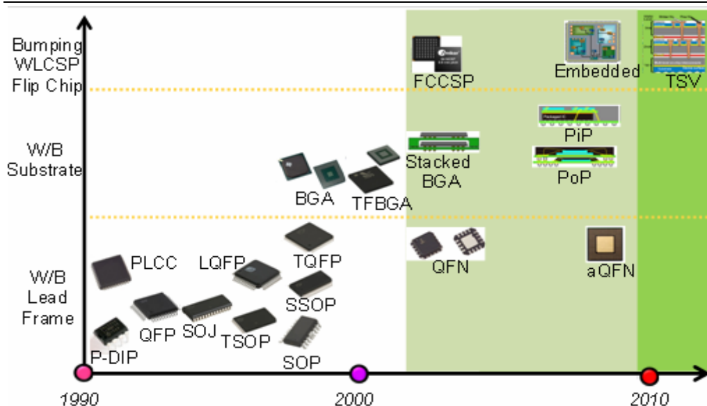
1990~2010 年封裝技術演進概況
