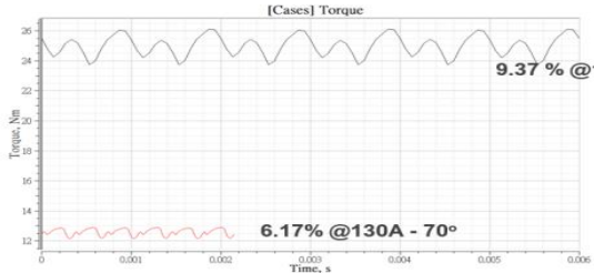
低轉矩漣波實現優異的NVH性能
