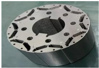
低轉矩漣波實現優異的NVH性能
