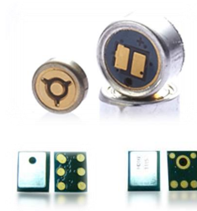
微機電麥克風/ 電容式麥克風
