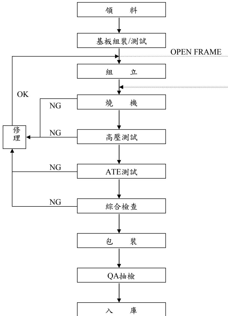
Power 生產流程圖
