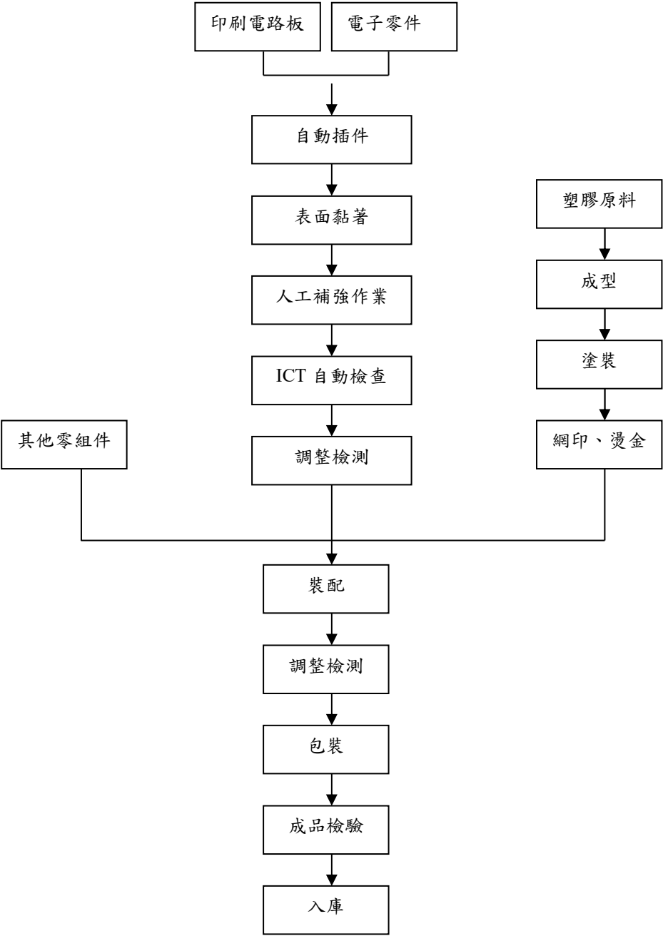
主要產品之產製過程
