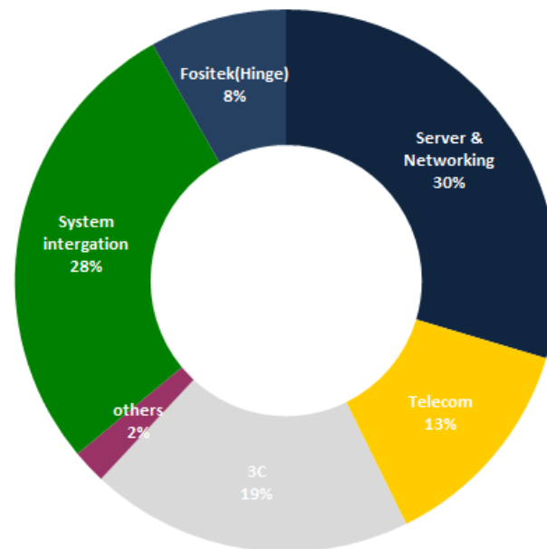
2022.Q4
