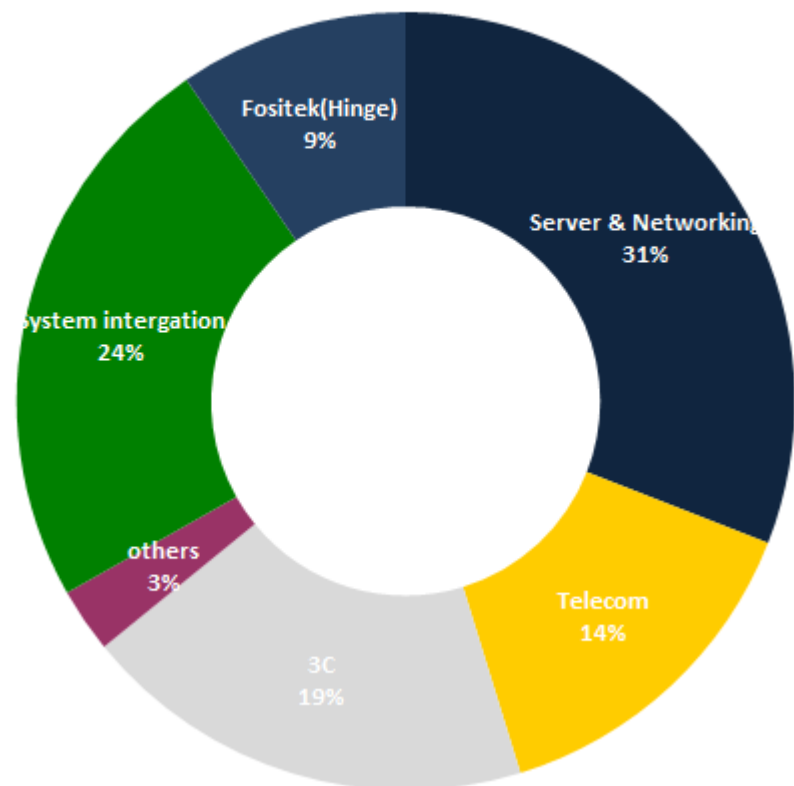
2023Y
