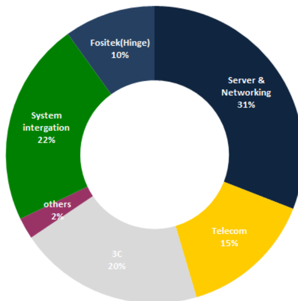
2023.Q3
