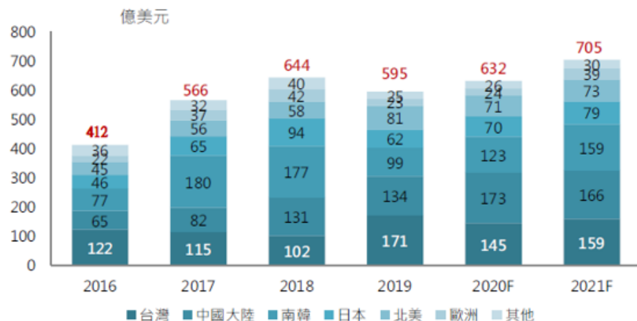
半導體製造設備銷售金額
