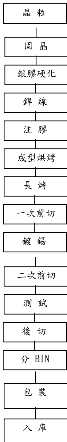
(1) Lamp 流程圖
