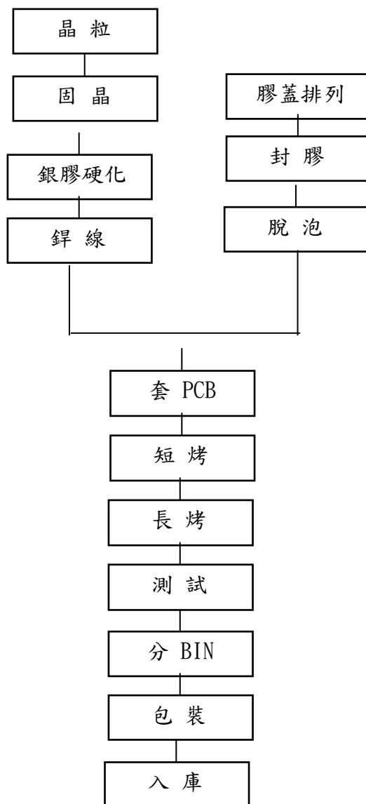
(2) Display 流程圖
