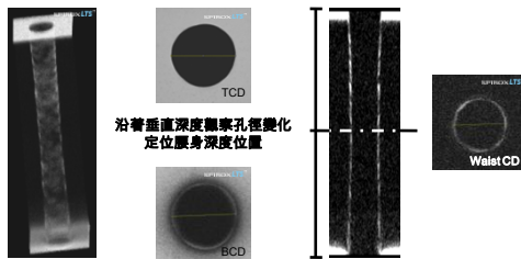
3D成像觀測TGV形貌
