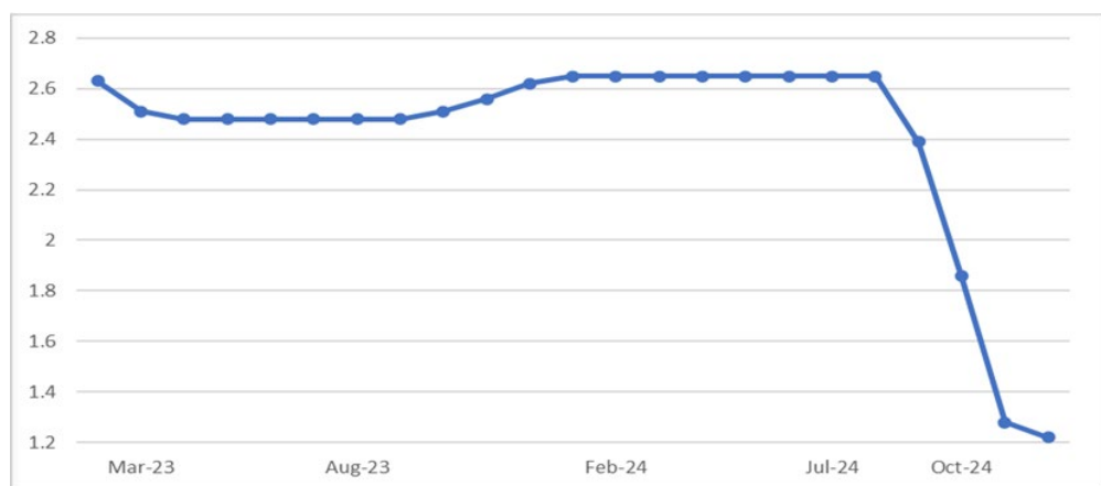
圖三、全球 NAND Flash 合約價格走勢
