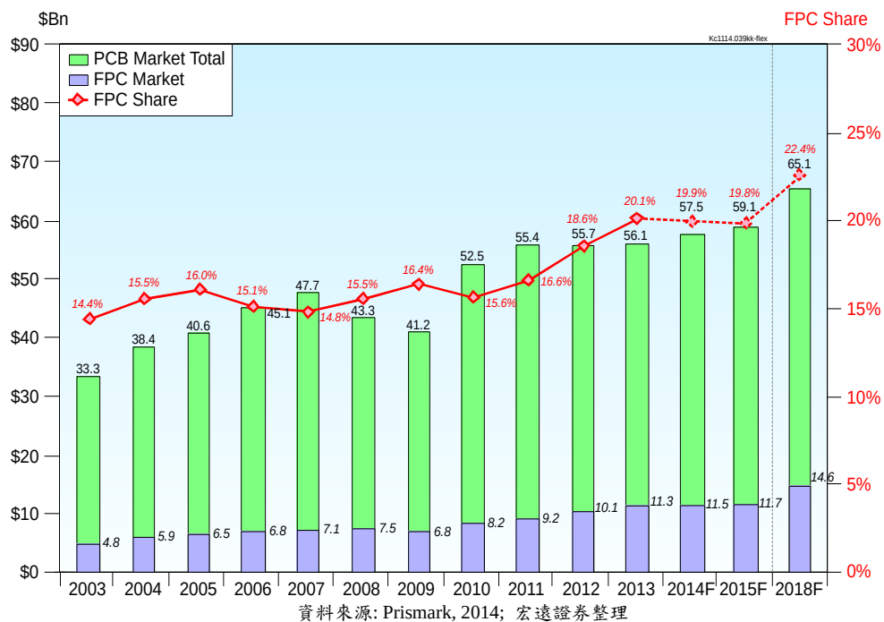
圖 1 印刷電路板市場成長趨勢
