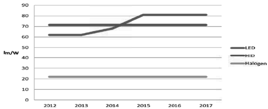
LED 頭燈與傳統光源頭燈發光效率變化
