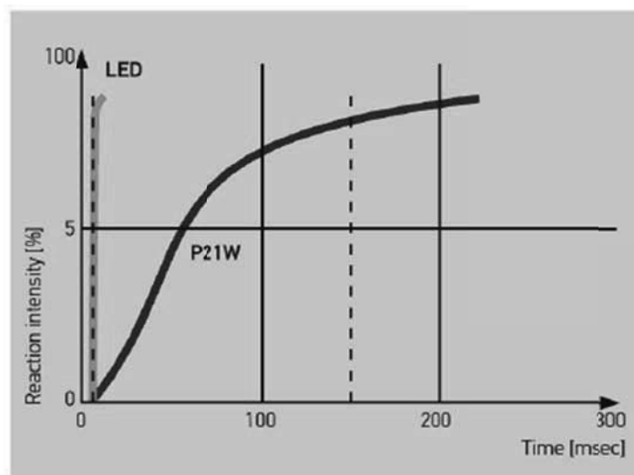
LED 與白熾燈泡反應時間比較
