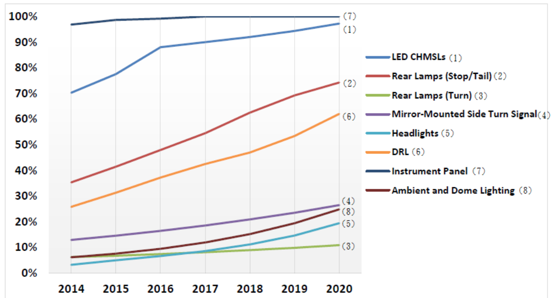
2014~2020 年全球 LED 車燈滲透率變化
