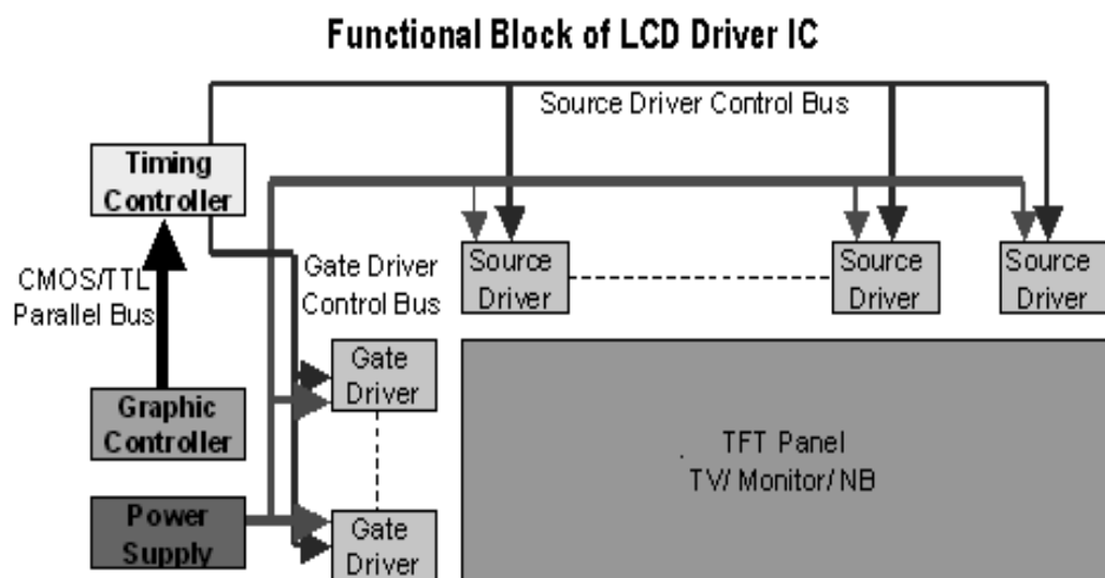
液晶顯示器基本驅動架構圖
