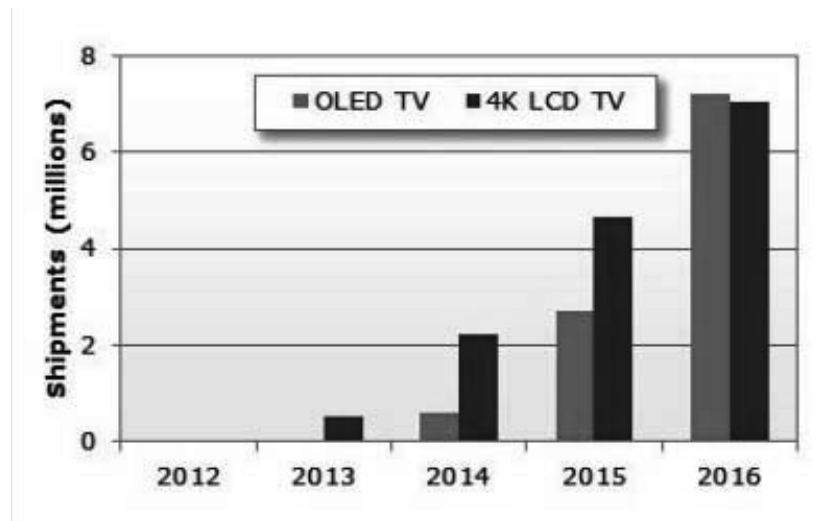
2012~2016 年 OLED 電視和 4K2K 液晶電視的出貨預測
