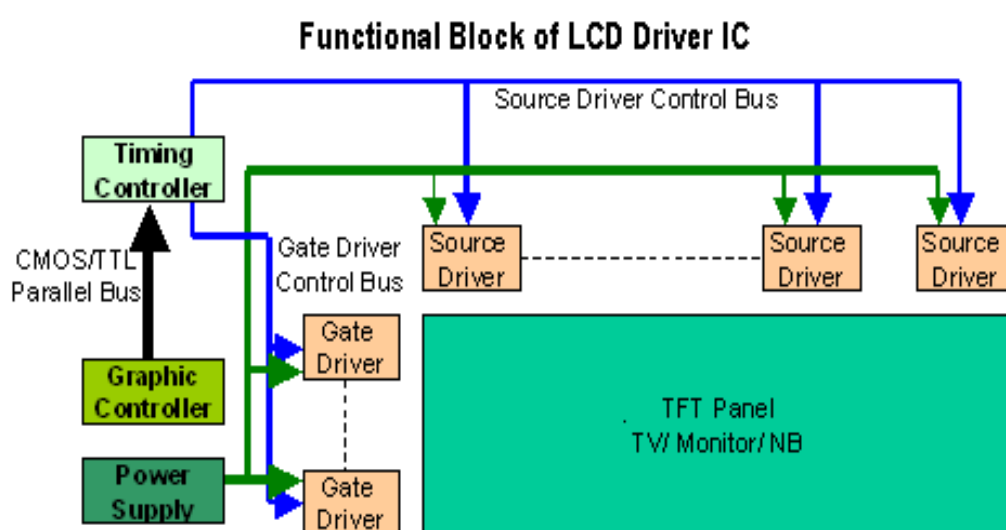
圖 5-1 液晶顯示器基本驅動架構圖
