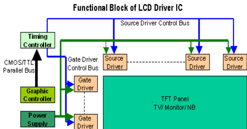
圖 5-1 液晶顯示器基本驅動架構圖
