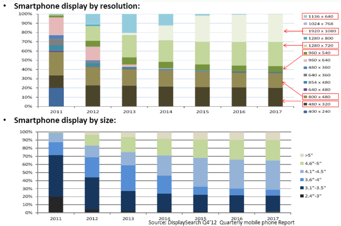
圖 5-4 智慧型手機面板朝大尺寸與高解析度發展
