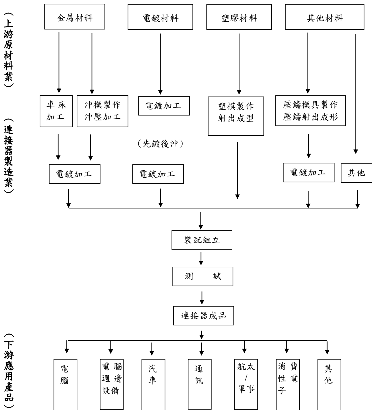
A.電子連接器之產業結構圖
