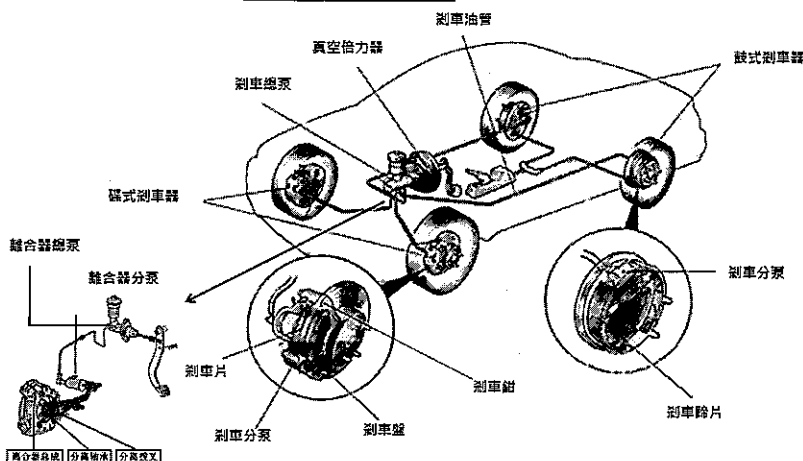
汽車剎車系統剖析圖
